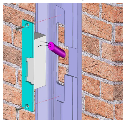
Wicket door
