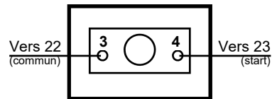
Boîte à bouton applique (BBA)
