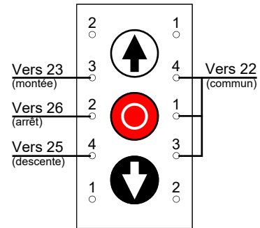
Boîte à 3 boutons applique (BBA3)
