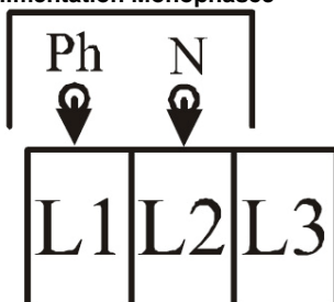
Alimentation Monophasée
