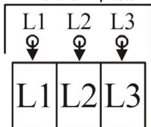
Alimentation Triphasée
