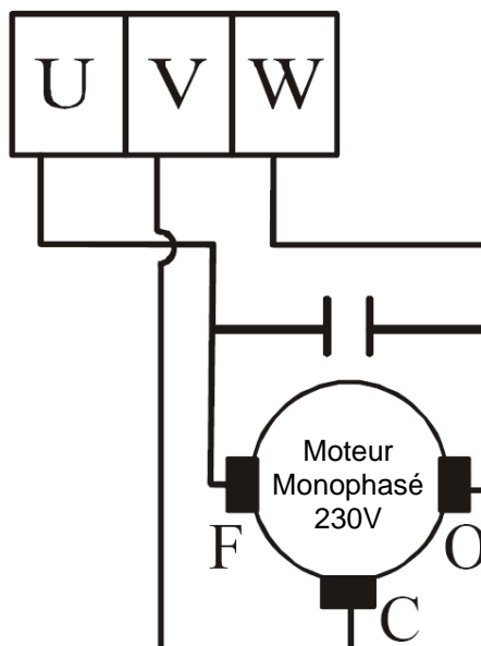
Alimentation Monophasée
