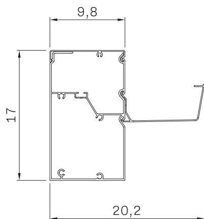
Profilé porteur (Périmétrique côté P avec gouttière)
