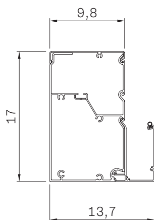
Profilé porteur (Périmétrique côté P avec gouttière et LED)
