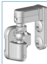
Gond n°4
