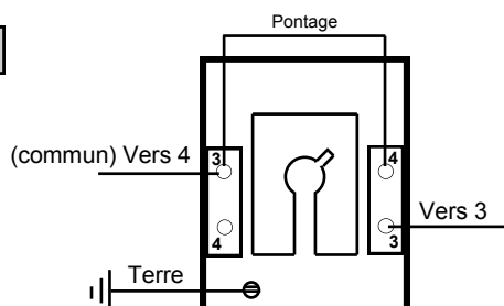
Boîte à clé (BCE2/BCA1)
