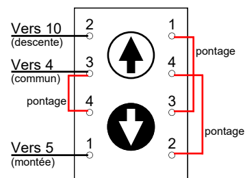
Boîte à 2 boutons applique (BBA2)
